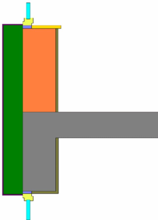
Рисунок Н.1 - Схематическое изображение вертикального разреза стены с теплоизоляционным фасадом в зоне расположения светопроемов с
