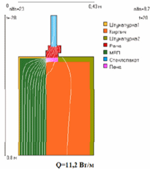
Рисунок Н.3 - Температурное поле узла конструкции, содержащего линейный элемент 2 Расчеты удельных характеристик других элементов проводятся аналогично и сведены в таблицу Н.2.
